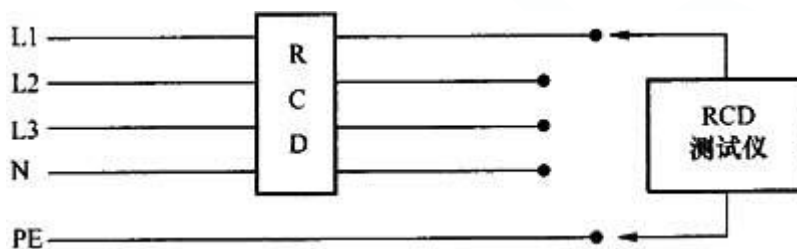
图1 测试方法
